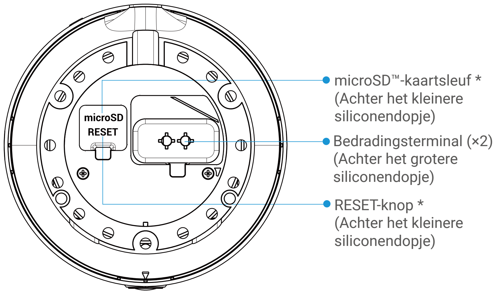
Onderaanzicht
