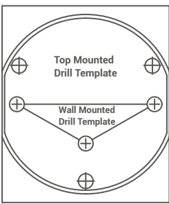
Boorsjabloon (×1)
